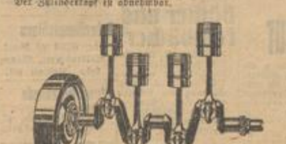
Im Innern der Danomag-Diesel-Zugmaschine...
