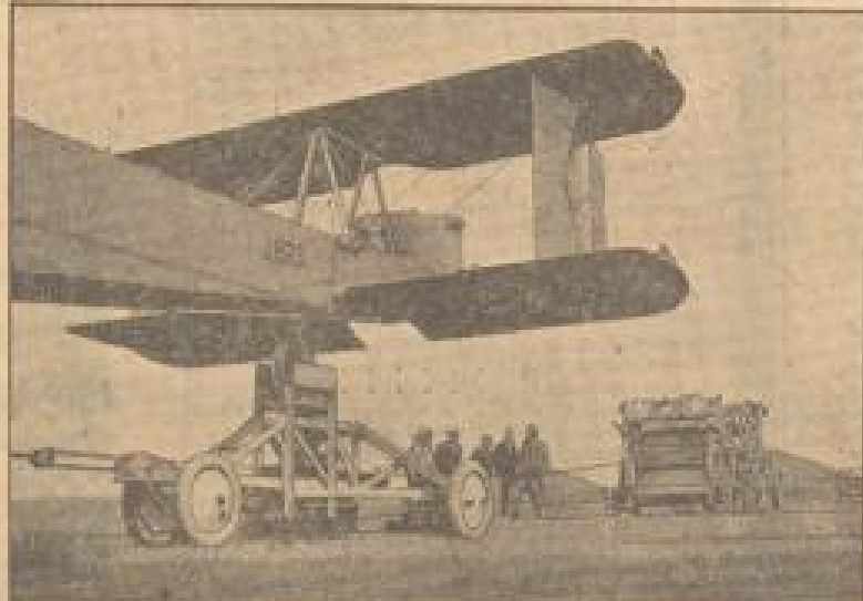
Englisches Bombenflugzeug beim Katapultstart. Oben: Das Flugzeug kurz nach dem Abflug. Unten: Der Schwanz des Flugzeuges ruht beim Abflug auf einem Startwagen, der auf Schienen läuft.
