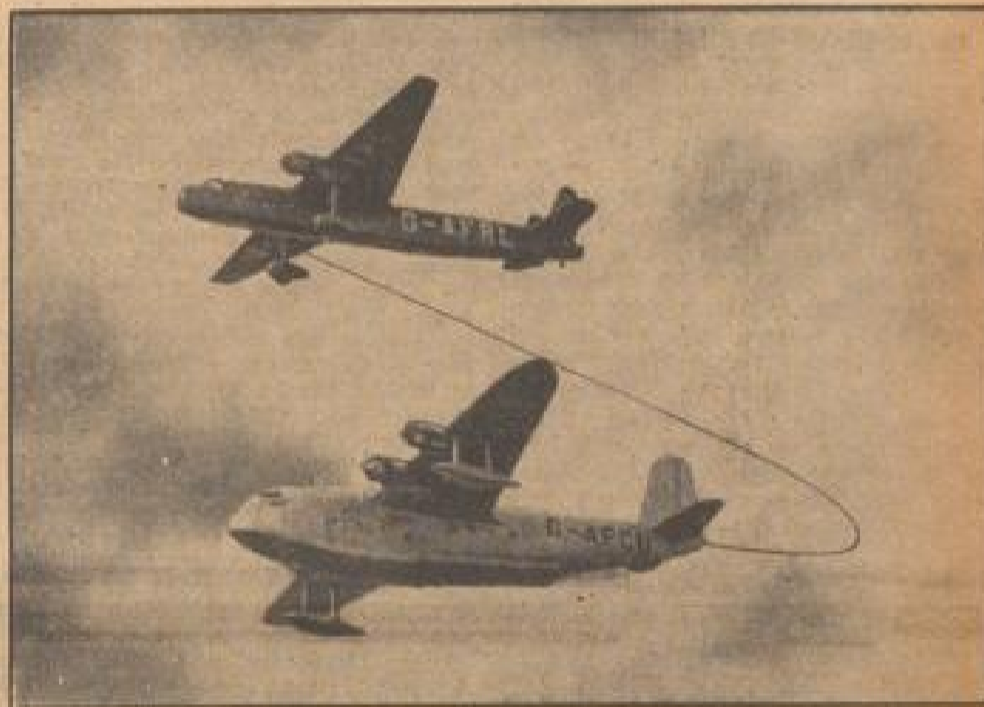
Ein fliegender Tank wurde bei einer englischen Transatlantiklinie über Southampton ausprobiert. Ein Bomber der englischen Luftwaffe trägt an das Flugzeug „Gaber“ während des Fluges einen 1000-galigen Tank. (Associated Press, London, N.Y.)
