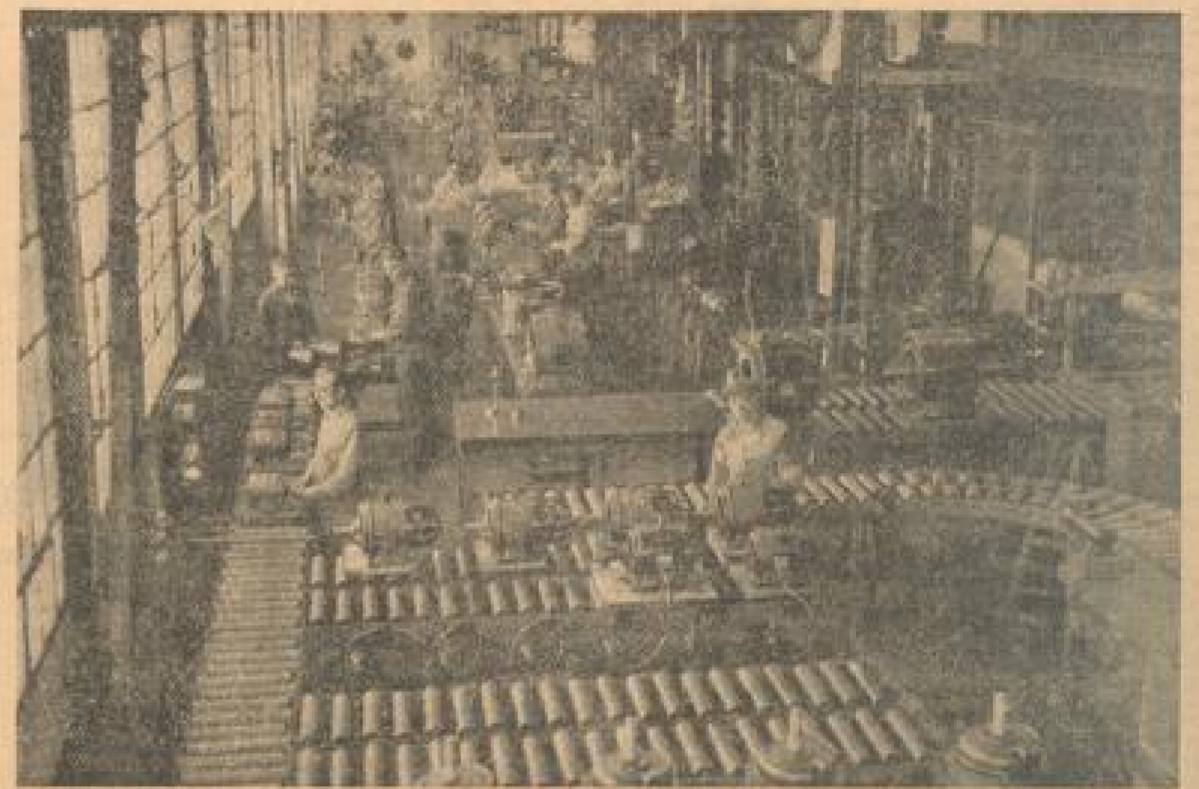
Ansicht der Montage-Halle für Kleinmotoren
