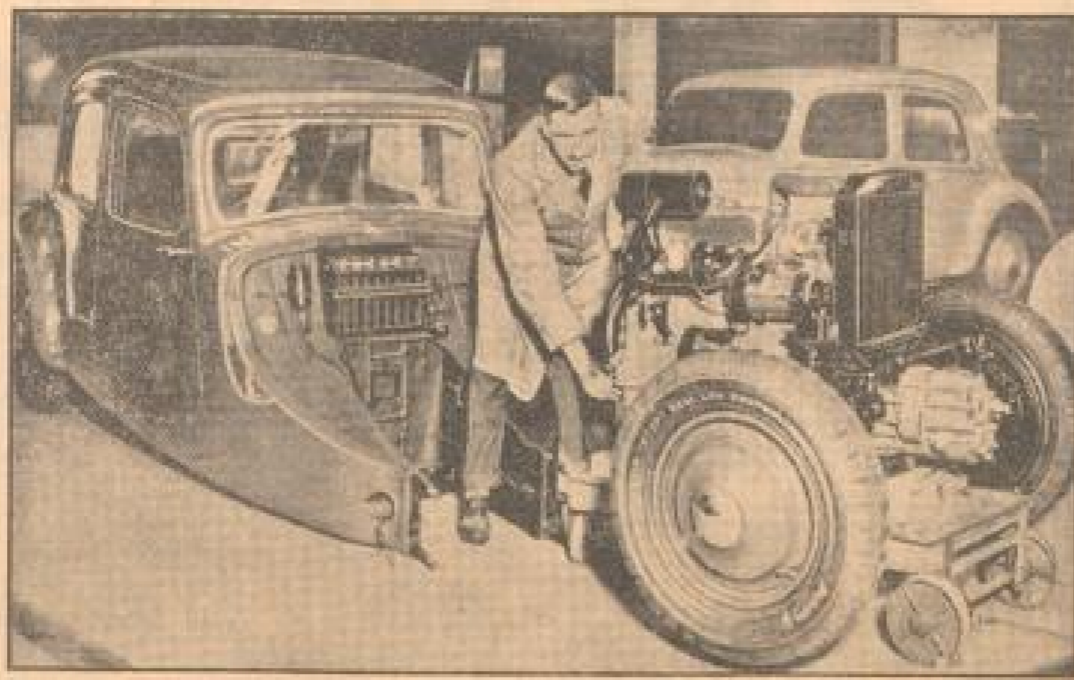
Eine vielbewunderte Neuerung auf der letzten in London eröffneten großen Olympia-Ausstellung ist dieses zerlegbare Auto...
