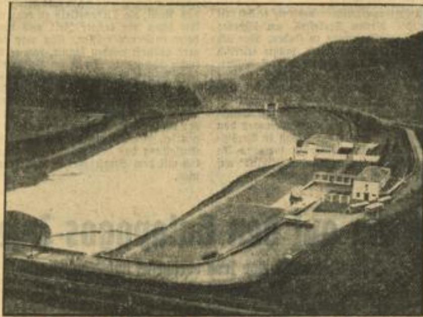
Eine der modernsten Staudämme Deutschlands, die Söfetsalperre im Harz. Ihr Hauptzweck ist es, das Gebiet zwischen dem Harz über Hildesheim bis nach Bremen mit Trink- und Brauchwasser zu versorgen.
