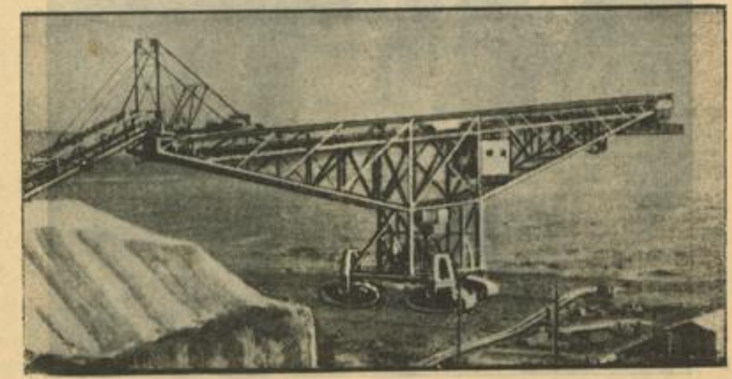
Auf einer rheinischen Braunkohlengrube kam die erste, von der AGW vollständig elektrisch ausgerüstete Abraumförderbrücke mit Raupenfahrwerk in Betrieb. Die drei das Bauwerk tra- genden Raupen haben die ungewöhnlichen Abmessungen von 9 Meter Länge, 3 Meter Höhe und 2 Meter Breite
