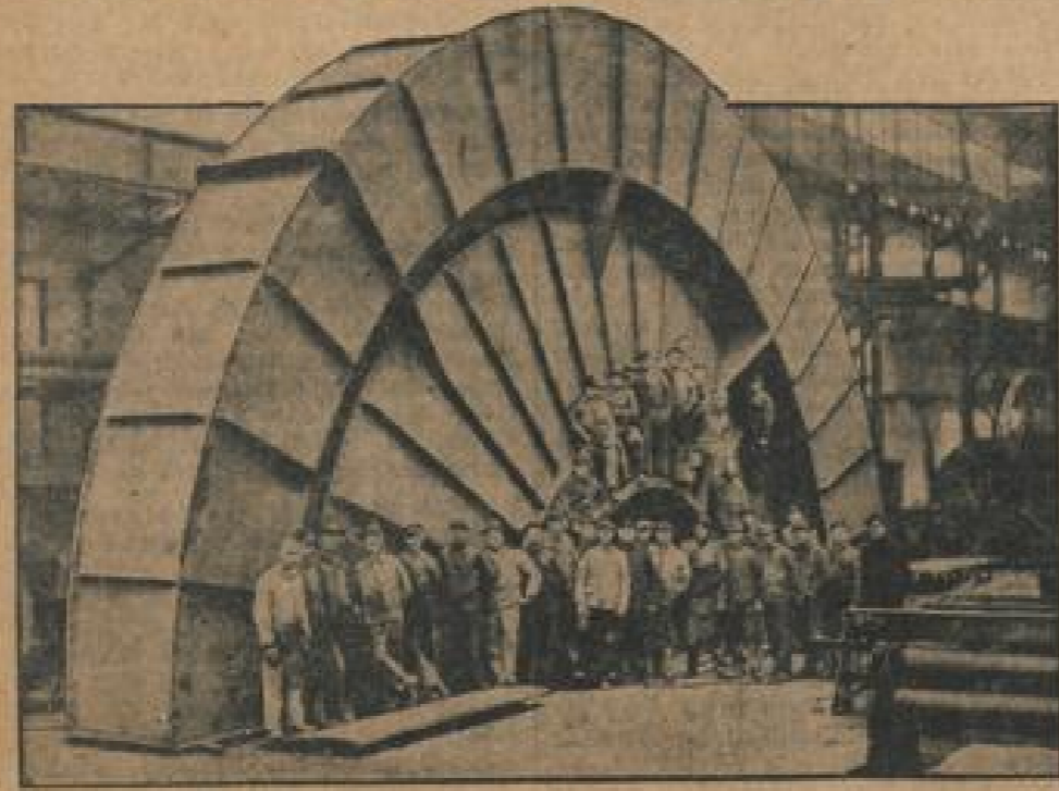
Meisterwerk eines Fabrikanten zeigt dem Reichs-Techniker, dem größten in der ganzen Welt, der hier fertiggestellt wurde. Das Modell hat einen Durchmesser von 10,5 Meter und vermag eine Leistung von 30000 PS zu leisten.
