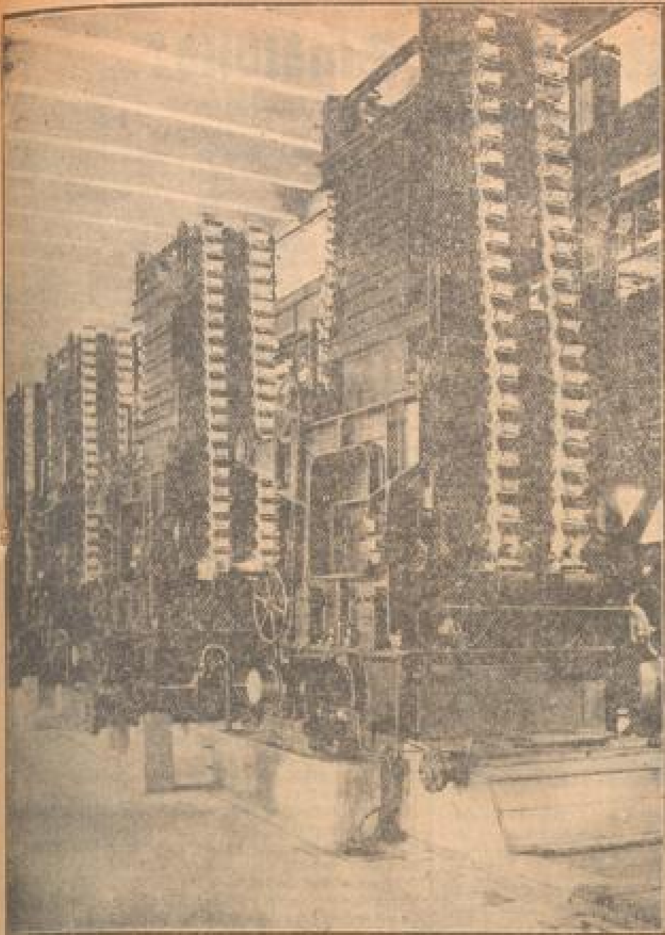
Reihe der großen Schleifer, die das Holz zerreiben
