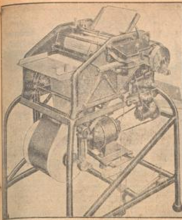
Neuzeitliche Vervielfältigungsmaschine
