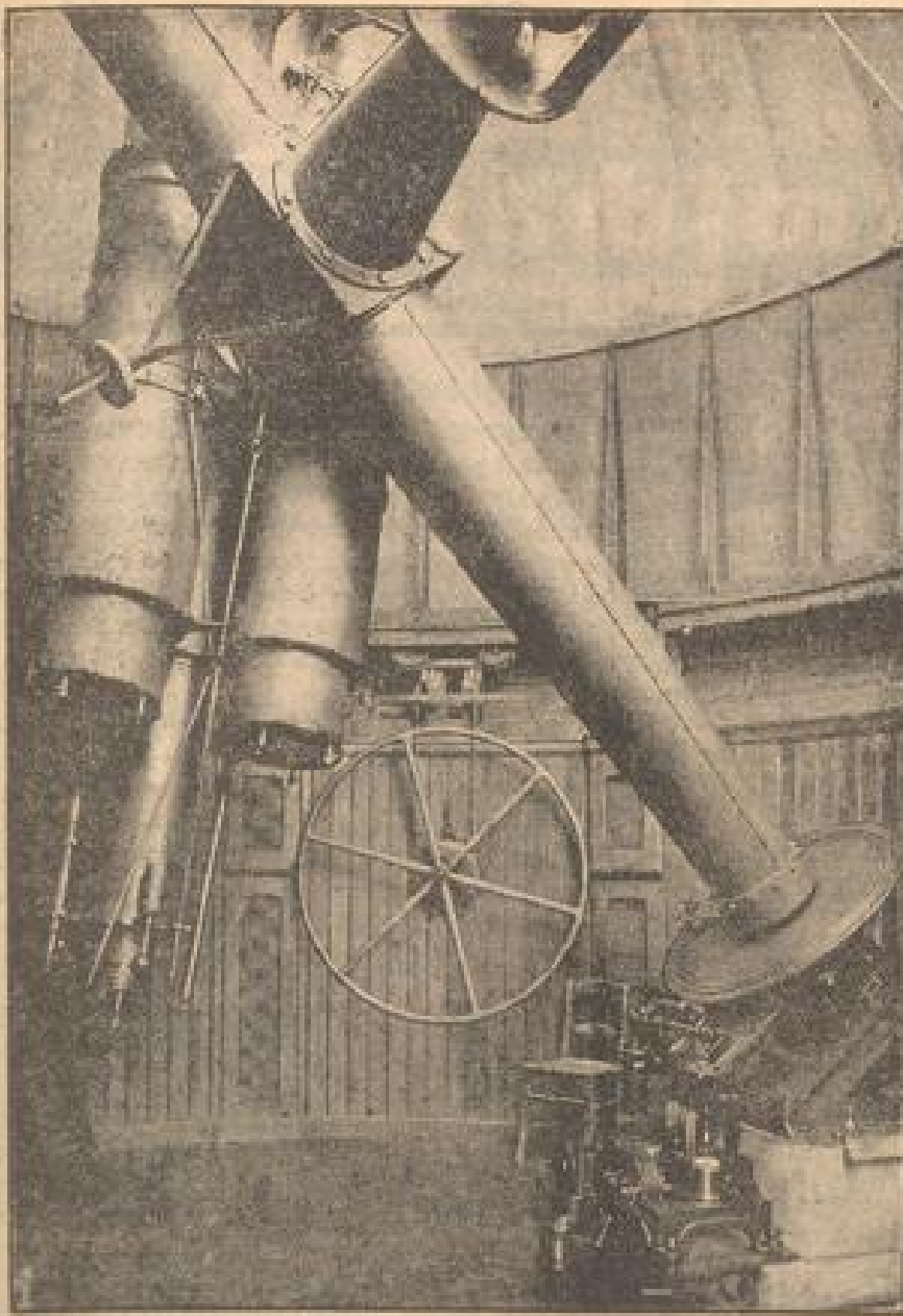
Das mächtige Himmelskanon: Das Heidelberger Bruce-Teleskop. Ein photographischer Doppelrefraktor.
