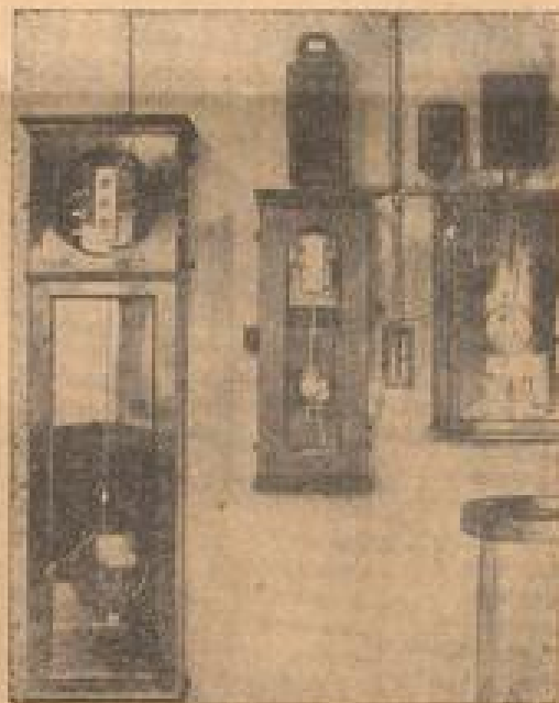
Das sind die wichtigsten Instrumente der Deutschen Seewarte. Die größte Getriebezeitmaschine der Welt (rechts). Mit Hilfe dieses außerordentlich komplizierten Apparates werden für jedes Jahr im voraus die genauen Zeiten von Ebbe und Flut für alle Plätze der Welt errechnet. — Links: Ein Teil des Signalgebers für das durch die Großfunkstelle Nauen ausgestrahlte Zeitsignal. Es geht zurück auf die Ermittlung der genauen Uhrzeit mit den Instrumenten des Instituts.
