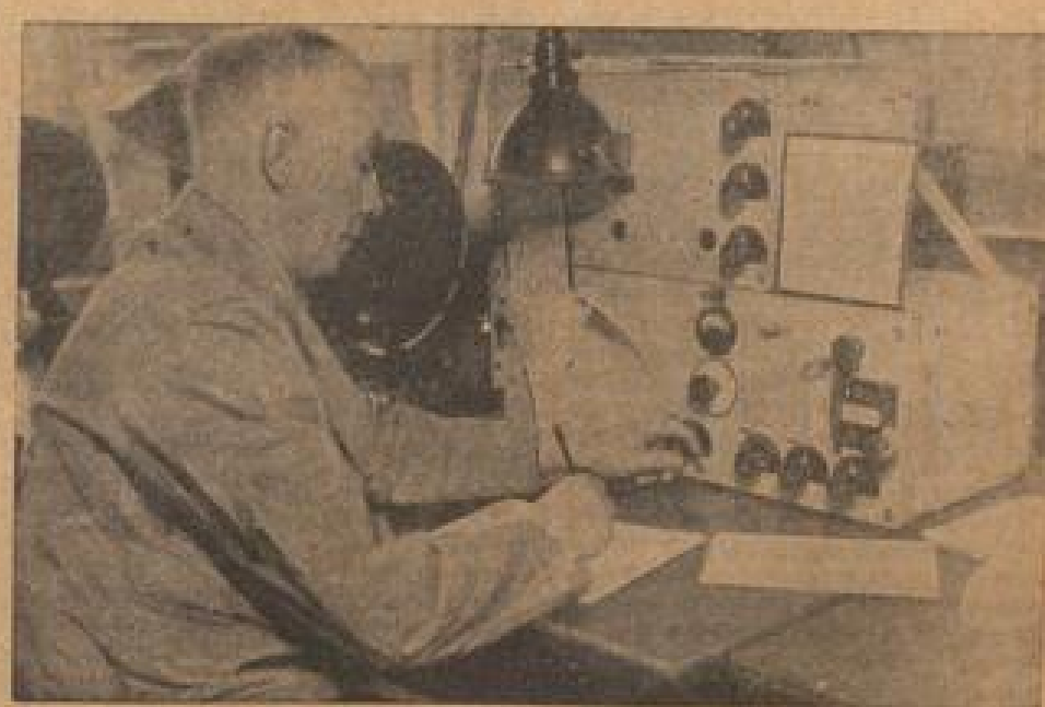
Wetter aus aller Welt! Die Deutsche Seewarte empfängt von zahlreichen Plätzen Mitteleuropas, der europäischen Meere und der Ozeane täglich Wetternachrichten. Die Aufnahme dieser Nachrichten erfolgt durch hochempfindliche Empfangsgeräte.
