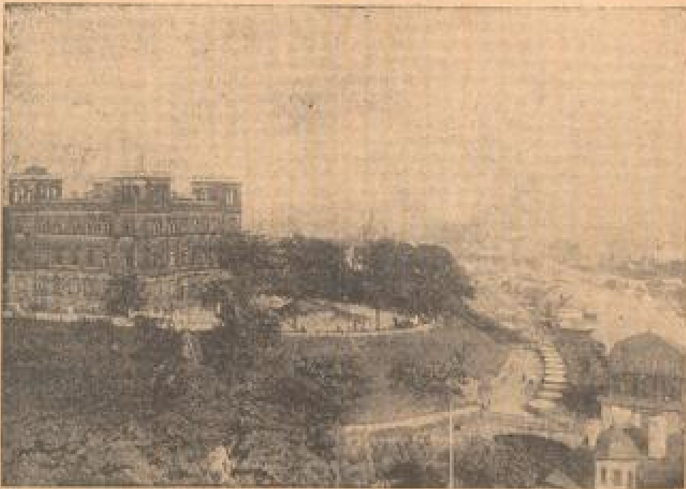
Auf dem Stützpunkt in Hamburg steht die Deutsche Seewarte. Man sieht es dem Gebäude mit der schlichten Fassade nicht an, welche Bedeutung es hat. Nur das Gewirr von Antennen und Masten verrät eine besondere Aufgabe. Hier wird die Zeit gemacht, hier werden die Geheimnisse des Wetters enträtselt und der weiten Ozeane.
