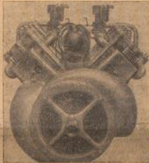
Luftgekühlter 8-Zylinder-Krupp-Vergasermotor
