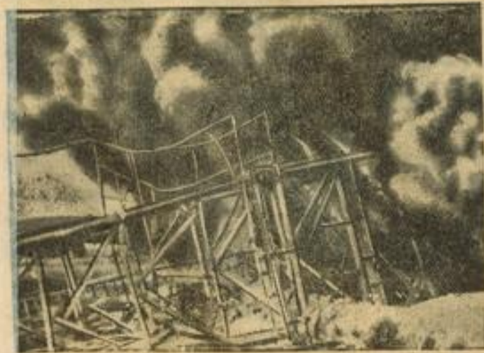
Der Erdölbrand bei Riechagen Blick auf die brennende Erdölquelle auf der Bohrung „Riechagen 22“; im Vordergrund der 40 Meter hohe eiserne Turm, der durch die Hitze zusammengestürzt ist
