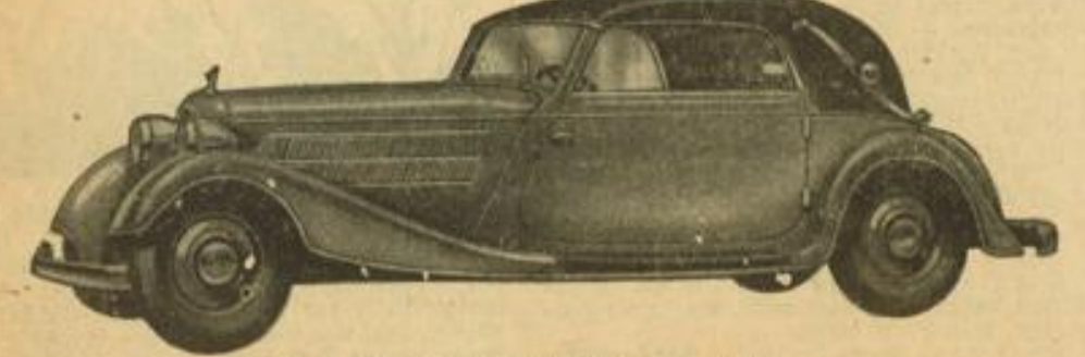
Auto Union-Audi-Front-Kabriolett, Luxus-Modell 50 PS-6-Zylinder-Motor mit hängenden Ventilen, Einzelschleifung, Frontantrieb
